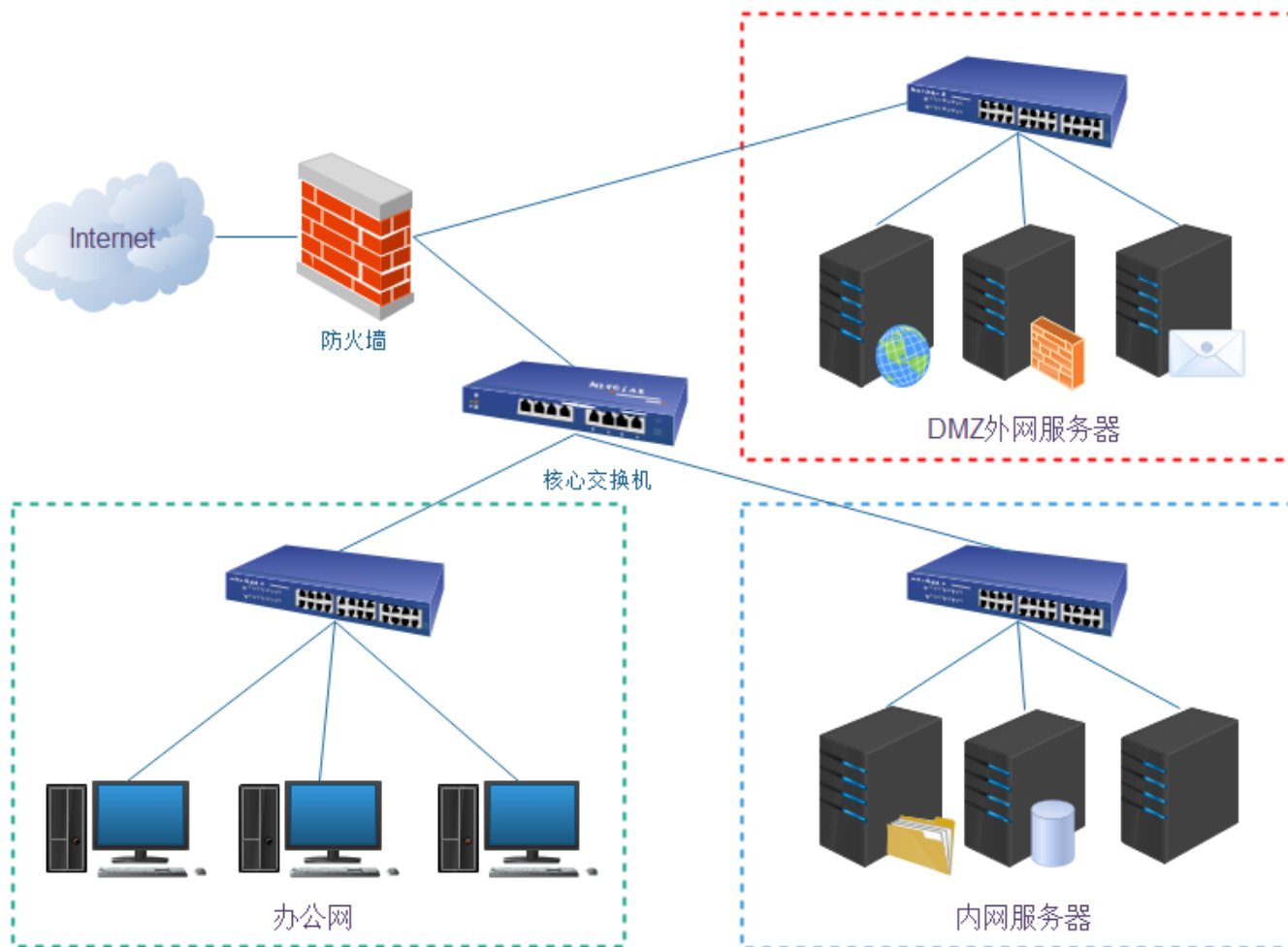
网络拓扑图
